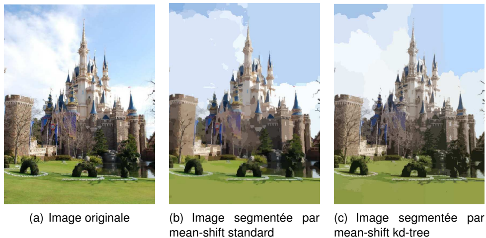
FIGURE 2.16 – Segmentation d’une image couleur de 2256 \times 3008 pixels.
