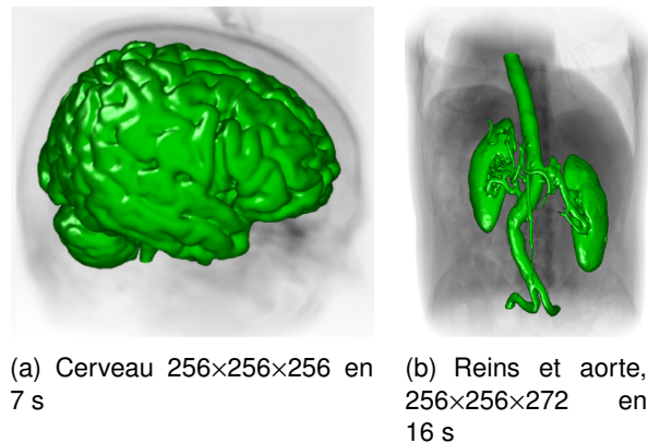
FIGURE 2.17 – Segmentation d’images issues d’examens IRM par la méthode des level set à bande étroite.
