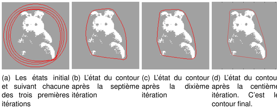
FIGURE 2.13 – Segmentation d'une image en niveaux de gris de 128 \times 128 pixels par algorithme dit du snake , dans sa version originale. Les paramètres d'élastictié, de raideur et d'attraction ont été fixés respectivement aux valeurs 5, 0.1 et 5.
