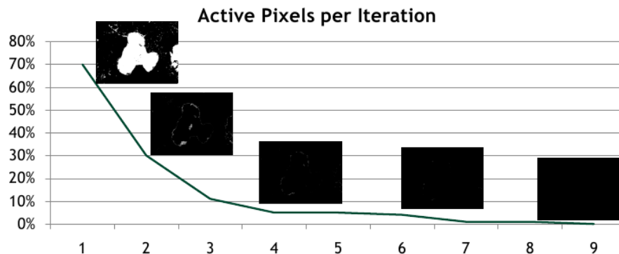
FIGURE 2.14 – Évolution du nombre de pixels actifs pour les itérations successives de l'implémentation de l'algorithme push-relabel de [79]. Les petites images montrent la localisation des pixels actifs après chaque itération, en blanc.
