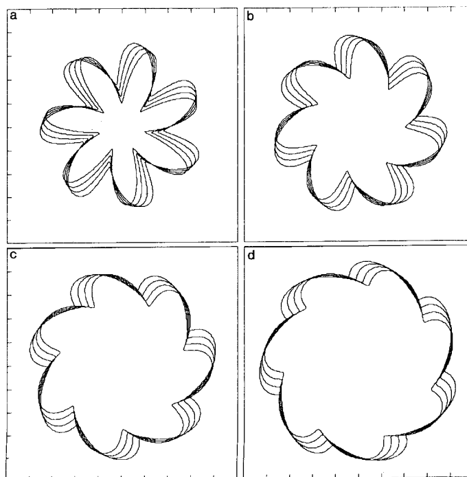
FIG. 7. Passive advection and propagation: F(K)=1+\text{Rotation} : (a) T=0.0, 0.03 (0.01) ; (b) T=0.03, 0.06 (0.01) ; (c) T=0.06, 0.09 (0.01) ; (d) T=0.09, 0.12 (0.01) .
