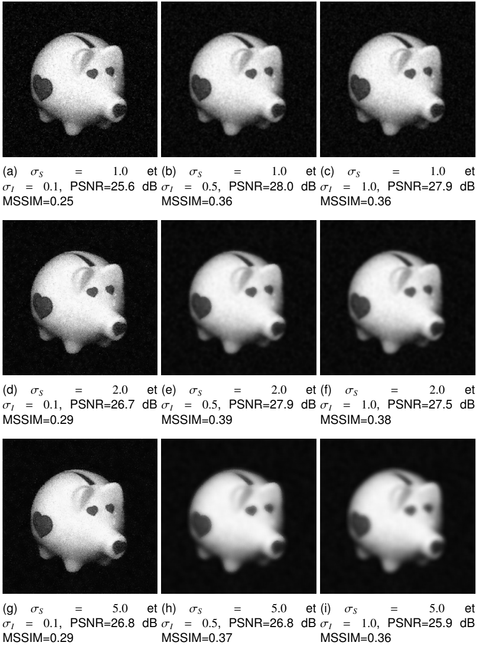
FIGURE 3.4 – Réduction de bruit gaussien par filtrage bilatéral de voisinage 5×5. \sigma_S et \sigma_I sont les écarts type des fonctions gaussiennes de pondération spatiale et d'intensité.
